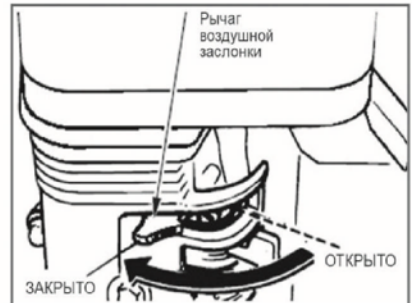
Установка рычага воздушной заслонки
